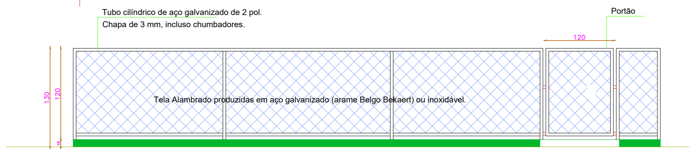
DETALHES ALAMBRADO 1/50
